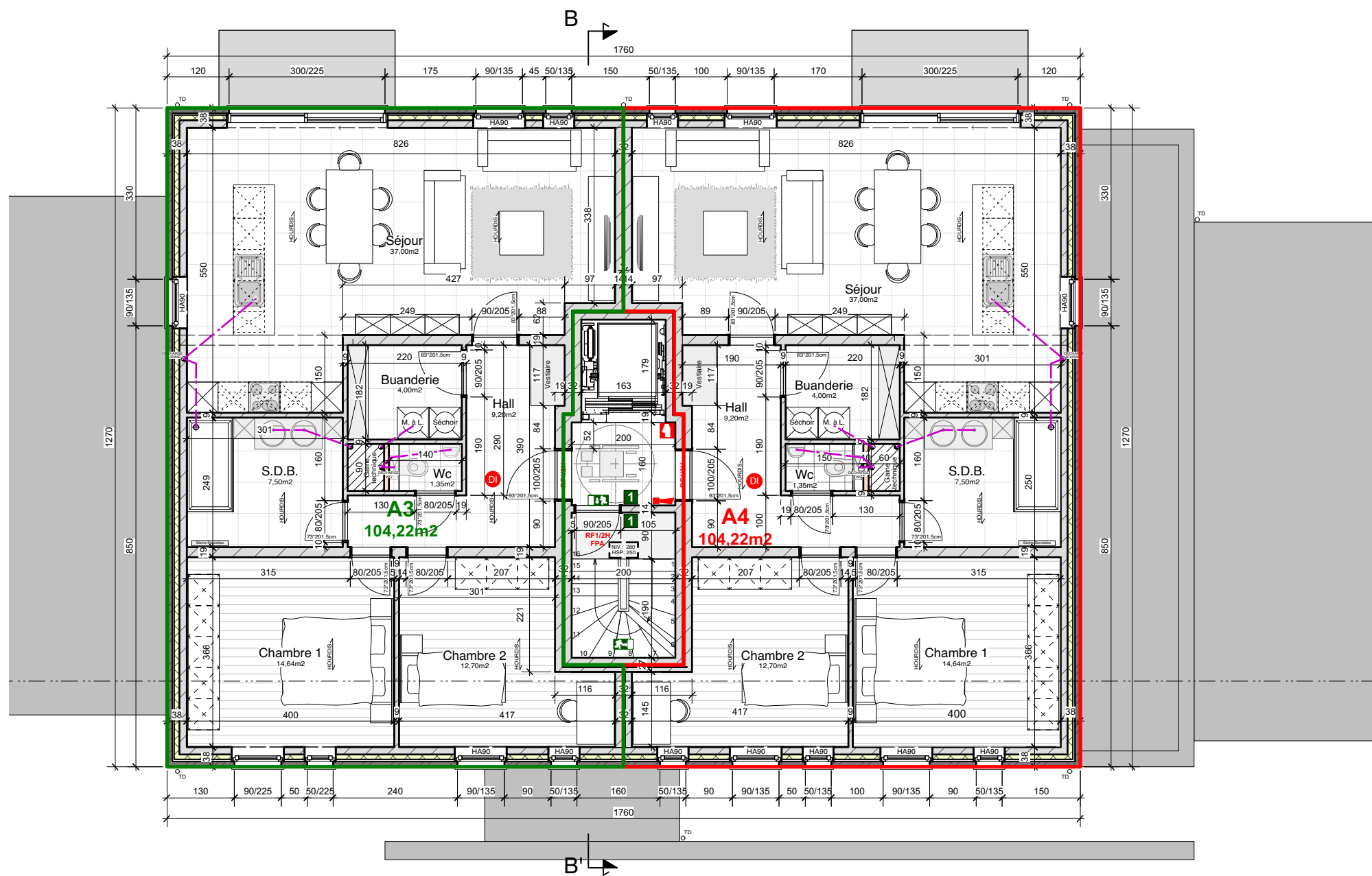
VUE EN PLAN DU PREMIER ETAGE - APPARTEMENTS
