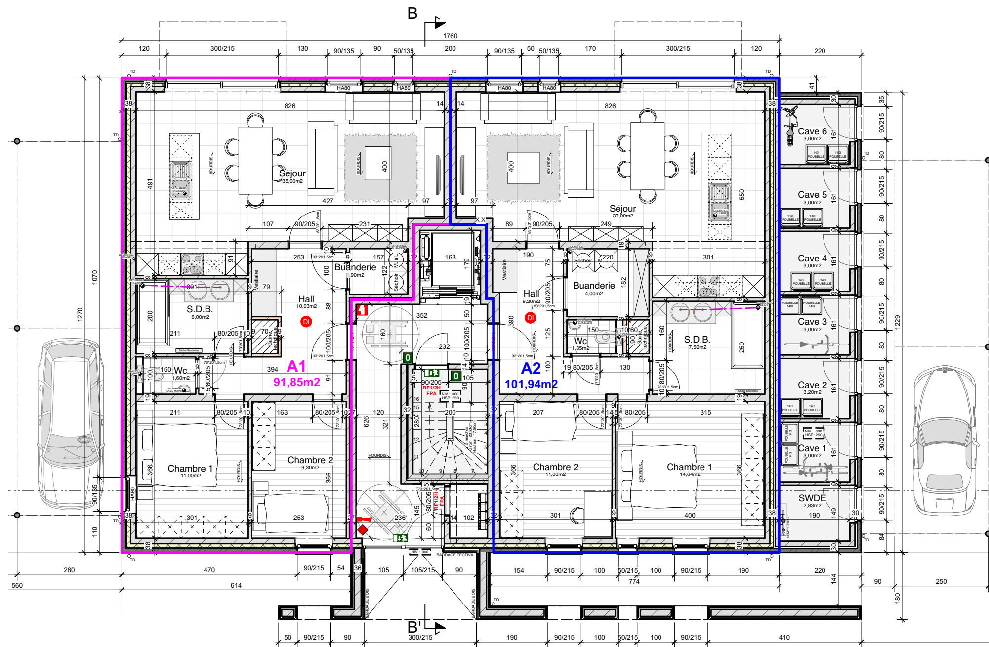
VUE EN PLAN DU REZ-DE-CHAUSSEE - APPARTEMENTS
