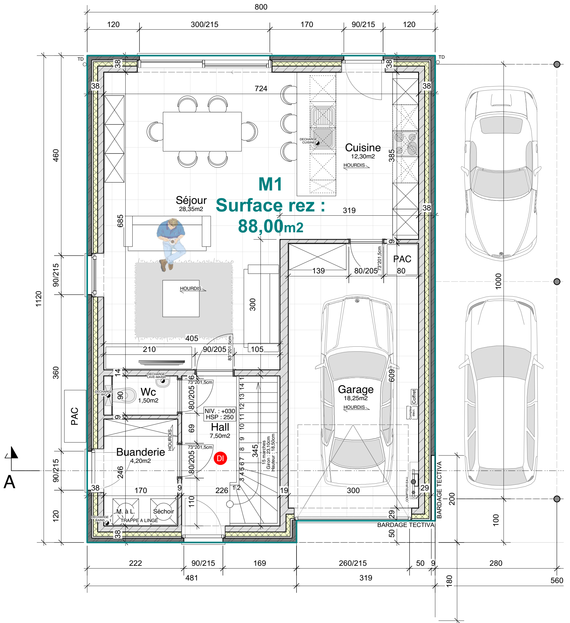
VUE EN PLAN DU REZ-DE-CHAUSSEE - MAISON 1
