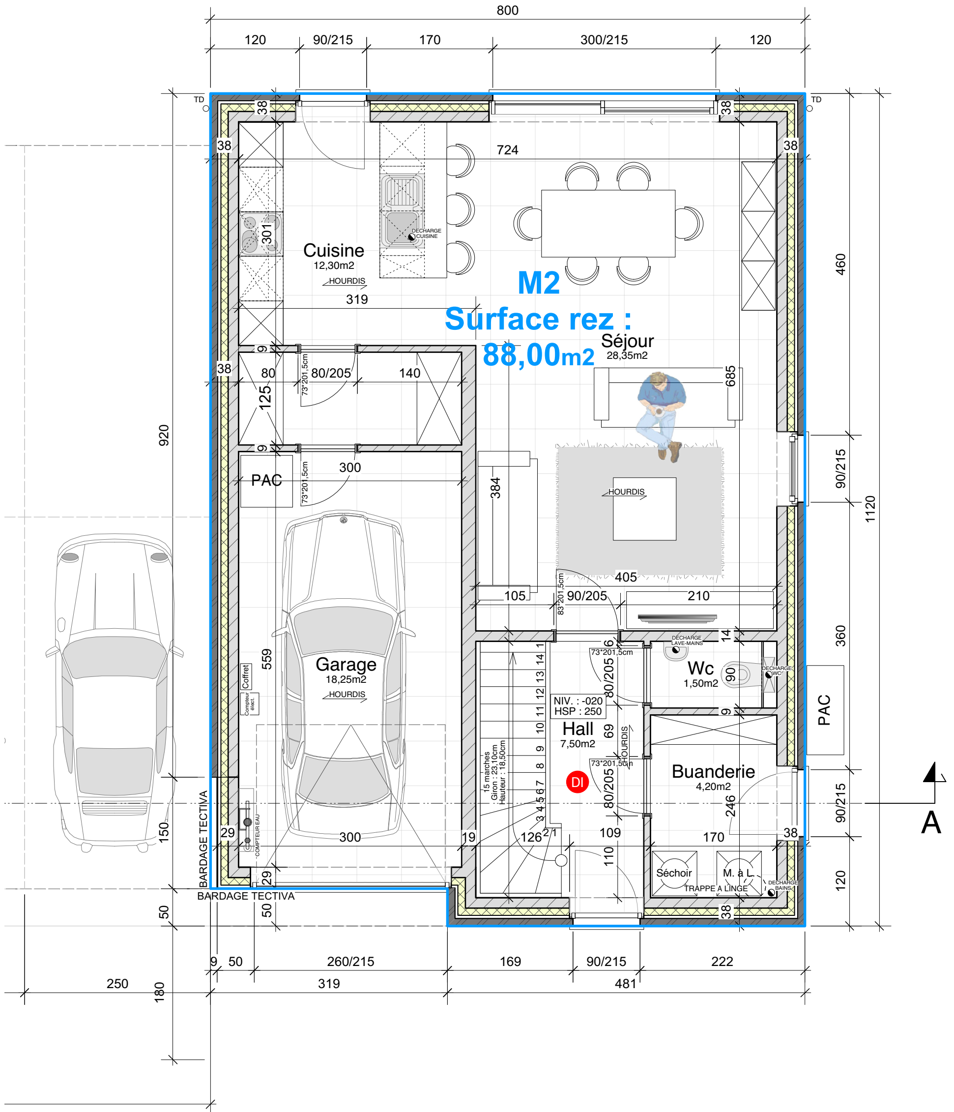
VUE EN PLAN DU REZ-DE-CHAUSSEE - MAISON 1
